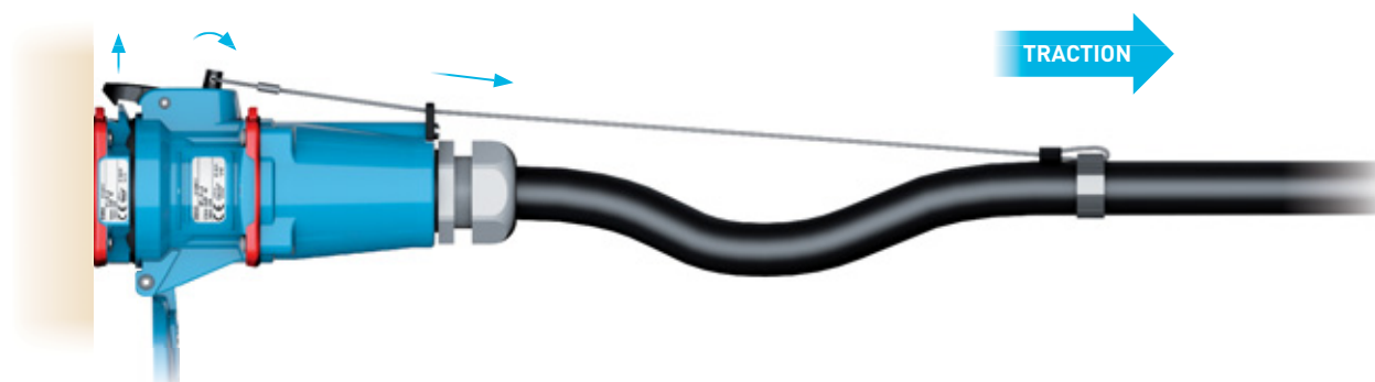
Étape 2 : la traction agit sur le câble électrique et le filin. Le crochet se lève progressivement.
