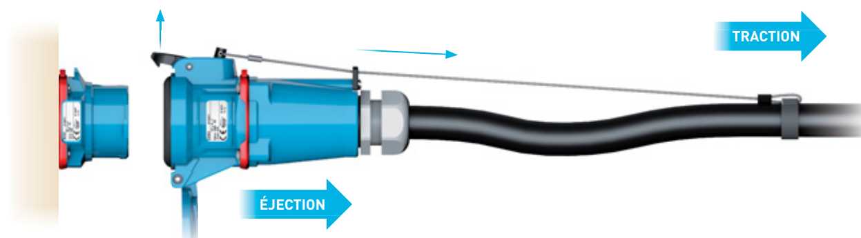
Étape 3 : le crochet est complètement relevé, entraînant l'éjection automatique du socle.
